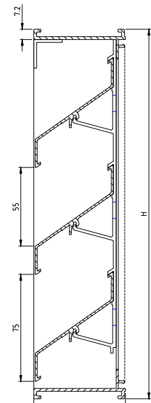
Cadre sans recouvrement n°451ZF
